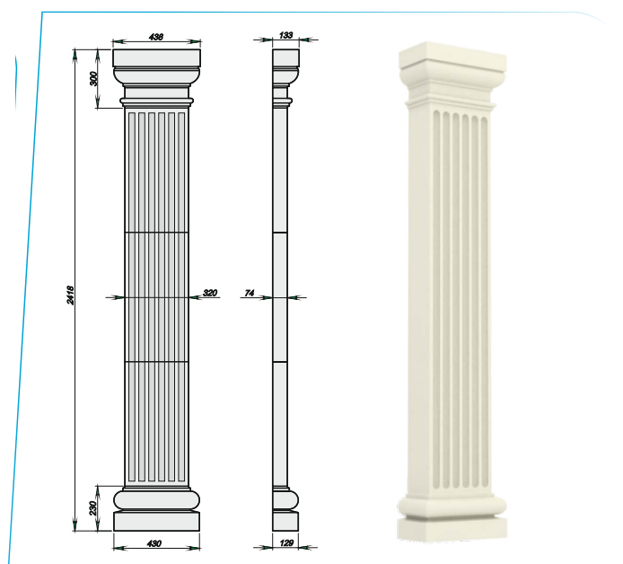
Пилястра_162
