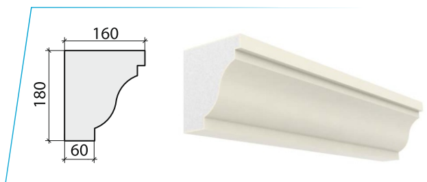
карниз_39
