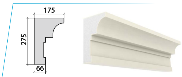
карниз_5
