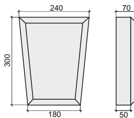
камень_150
