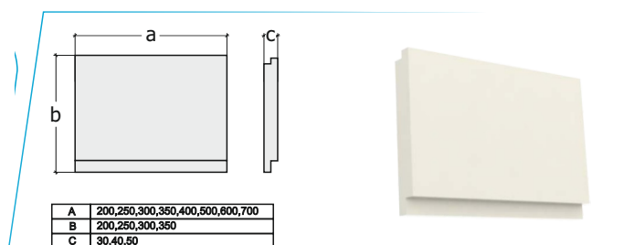
Руст_142
