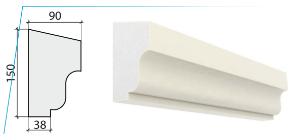
карниз_69
