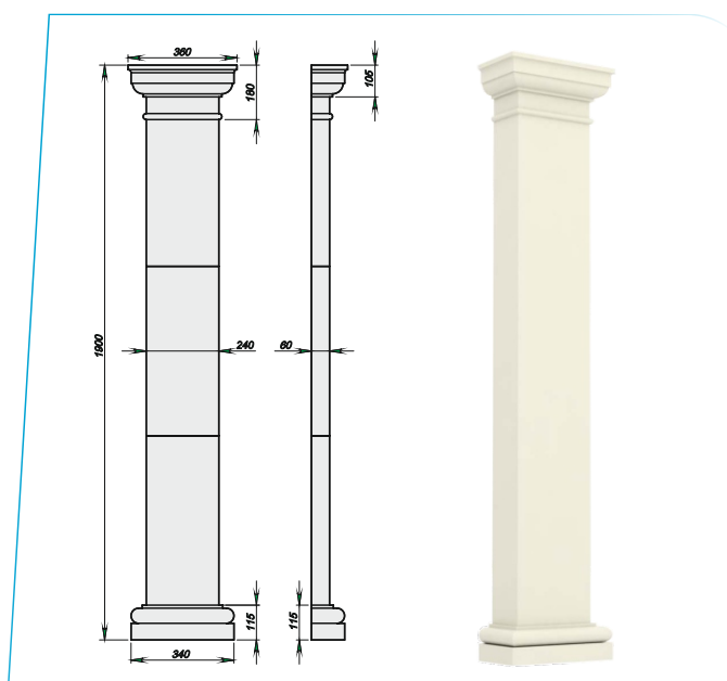
Пилястра_161
