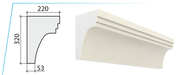
карниз_33
