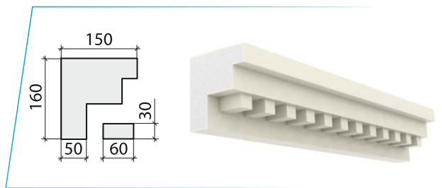
карниз_37
