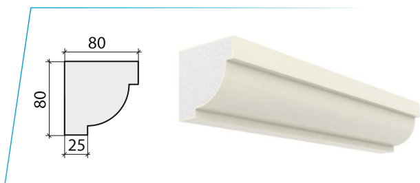
карниз_53
