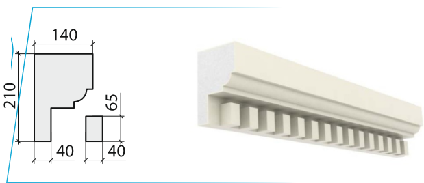
карниз_80
