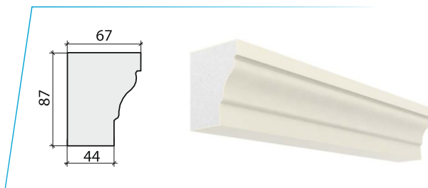
наличник_117
