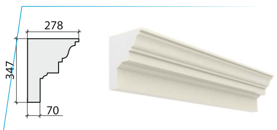
карниз_73
