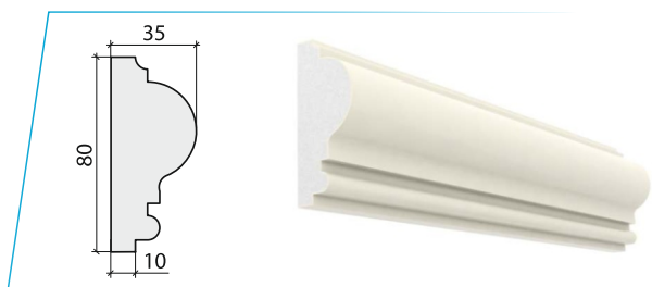
наличник_111
