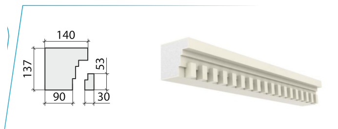
карниз_84
