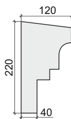
карниз_94
