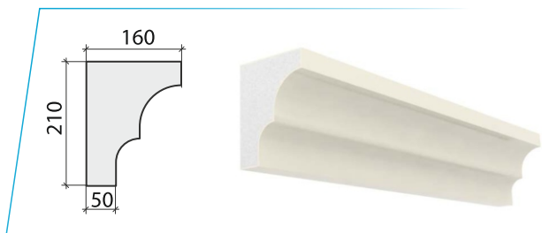
карниз_87
