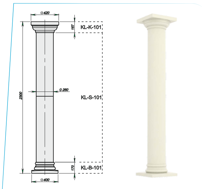
Колонна_159
