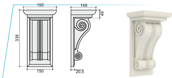
кроншт_145
