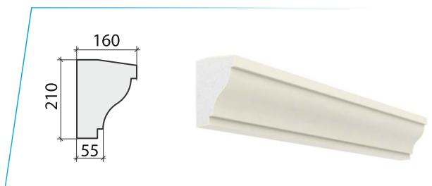
карниз_89
