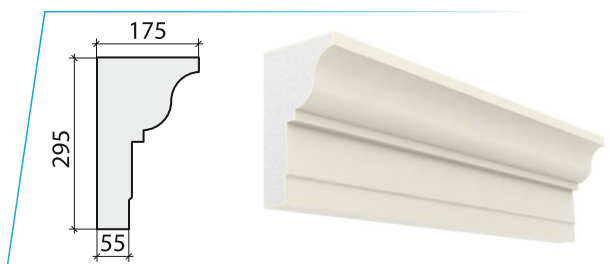
карниз_57
