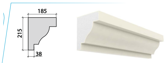
карниз_6
