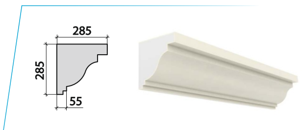
карниз_7
