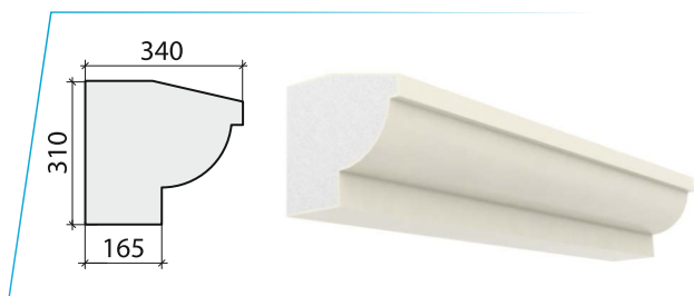
карниз_31
